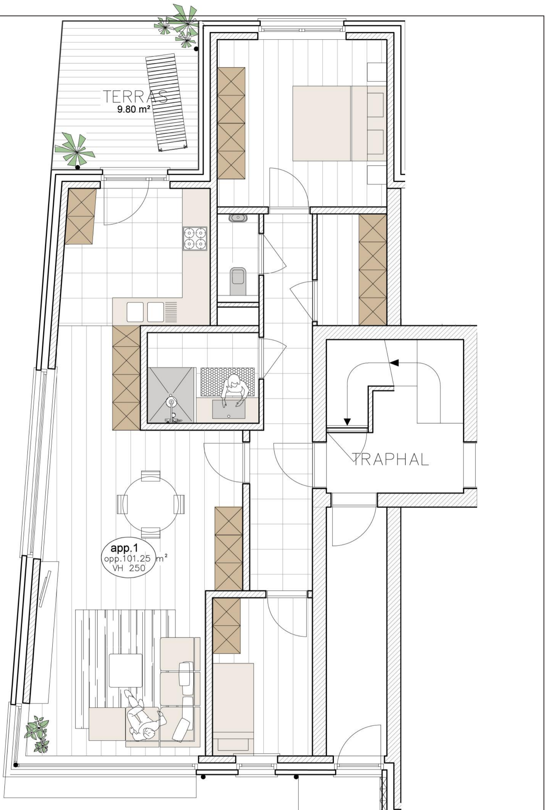
Gelijkvloers App. 1 Schaal 1/50 Opp. appartement. 101,25 Opp. terras 9,5
