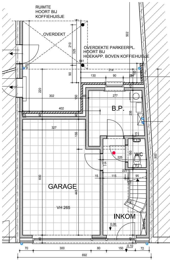
PLAN GELIJKVLOERS
